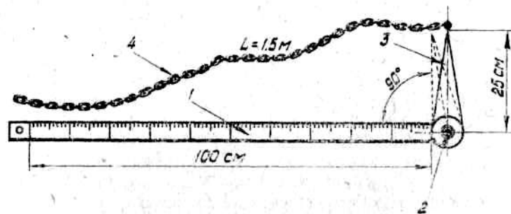
Рис. 2. Ледомер.
