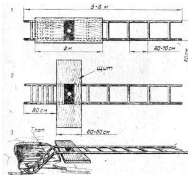
Рис. 10. Спасательная лестница № 2.
