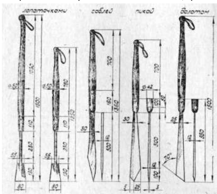
Рис. 1. Виды пешни.
