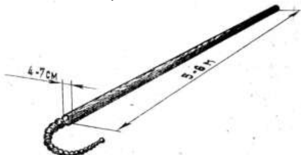
Рис. 8. Спасательный багор.
