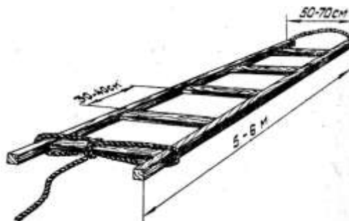
Рис. 9. Спасательная лестница № 1.
